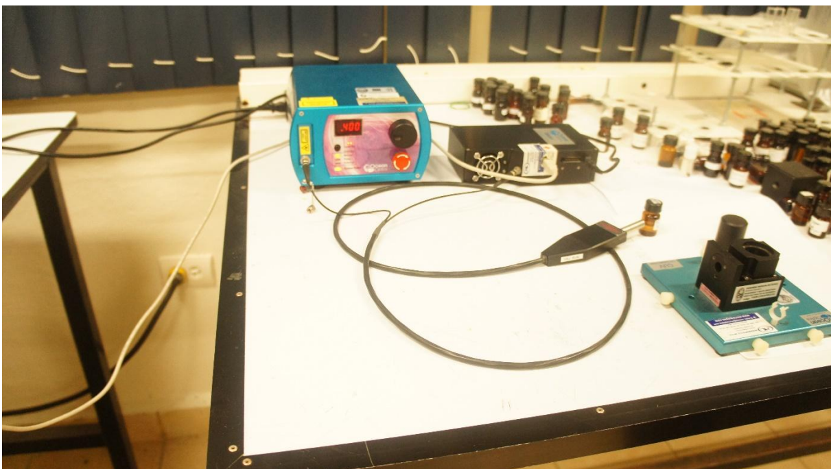
Espectroscopia Raman
